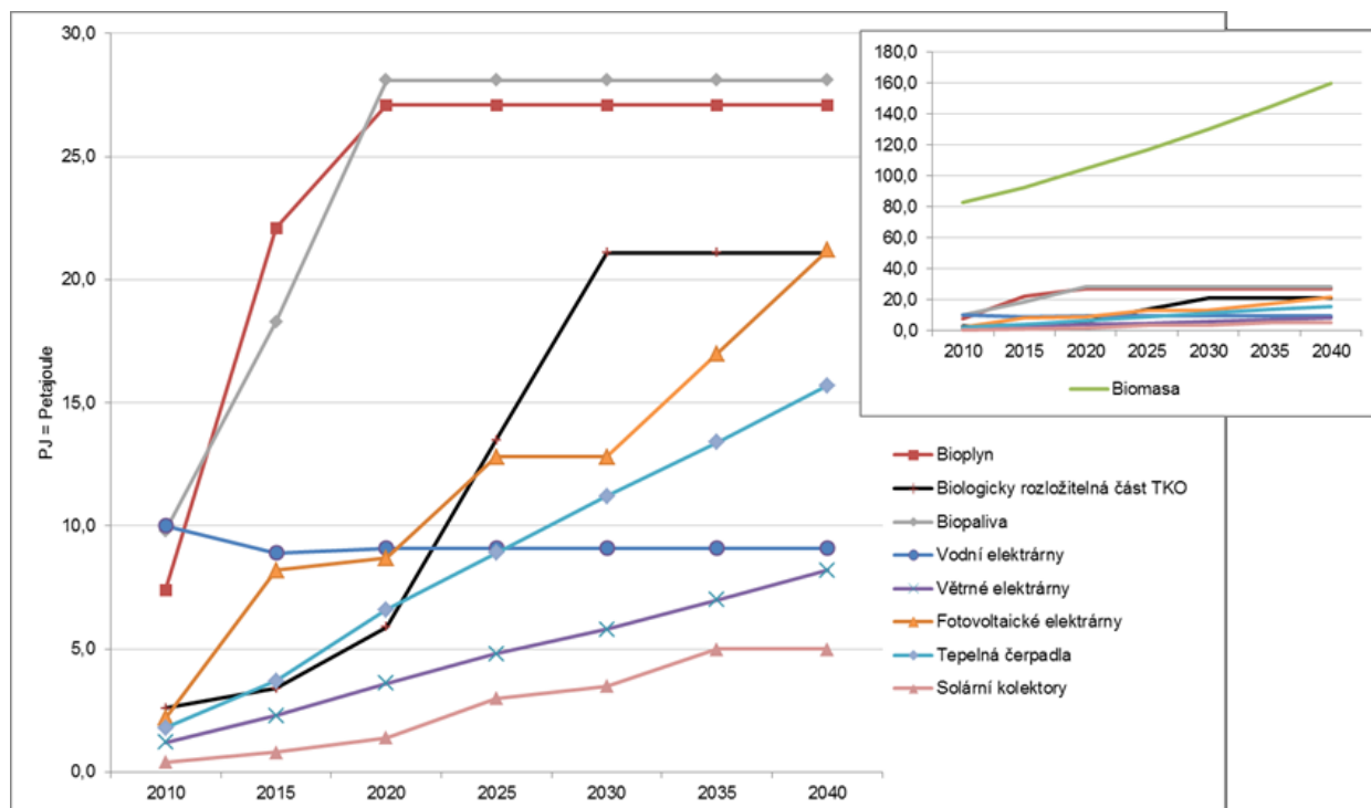
Graf č. 6 – Vývoj jednotlivých OZE na primárních energetických zdrojích v ČR v letech 2010–2040 podle optimalizovaného scénáře aktualizované SEK
